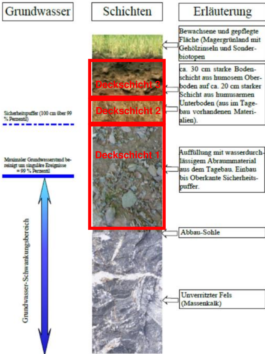
Abb. 1 Schematischer Aufbau der zukünftigen Deckschichten. Quelle: BUND 2021, verändert
